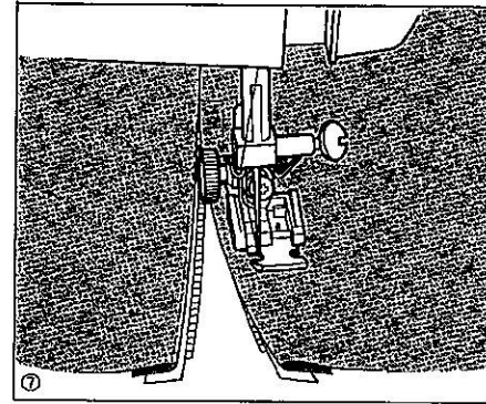
⑦ファスナーのスライダーを押えの向こう側にずらし、押えをおろして残りを縫う。
