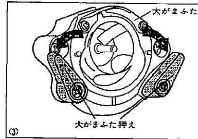
③大がまふた押えを左右にひらき大がまふたをはずす。
