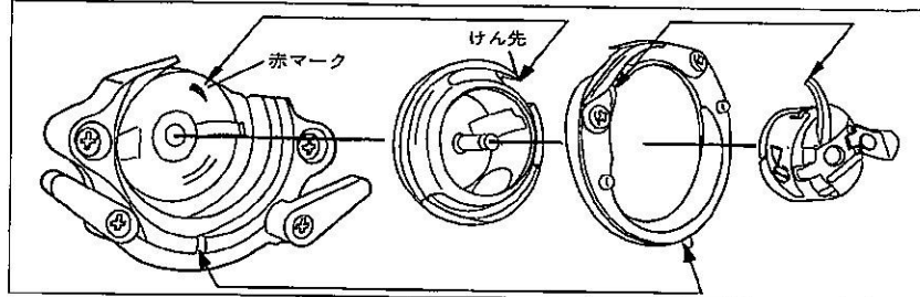
①赤マークに中がまのけん先を合わせてさしこむ。
