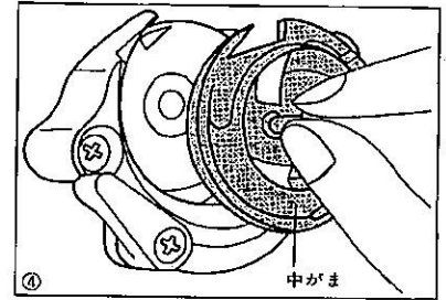
④中がまをはずす。
