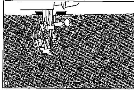
①あき止まりまで地縫いをし、縫いしろを割る。ファスナーのむしが見えないように0.1cmくらいかぶせて打ち合わせ、折り山から0.5cmはなしてあき止まりに向かって縫う。
