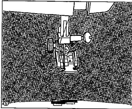
⑤押えを右側によせ、押え裏の左のみぞにファスナーのむしを合わせ、押えをおろす。基線ダイヤルを「左」よりやや中にセットし、針が押えの針穴いっぱいにおりるのを確かめて縫う。
