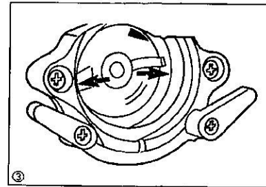
③矢印の部分にミシン油を1～2滴注油し、布切れで軽くふきとる。
