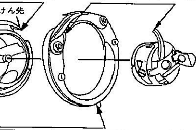
②大がまふたの突起を大がまの穴に合わせてはめこむ。
