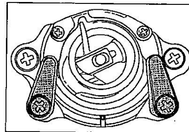
③左右の大がまふた押えをとじ、最後にボビンケースをとりつける。
